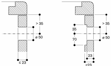
Installation af betjeningsgreb, plan montering
