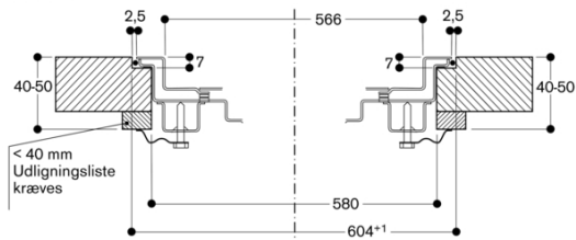
Tværsnit
