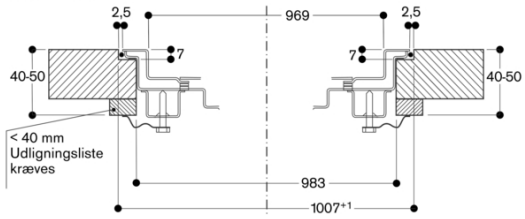
Længdesnit
