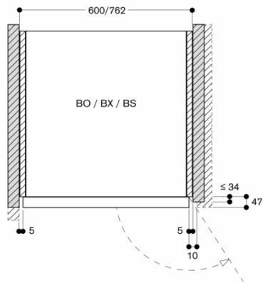
Tværsnit af luftindtag ved dørrammer
